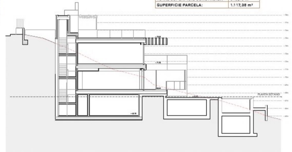
SECCIÓN A-A' 1:100
