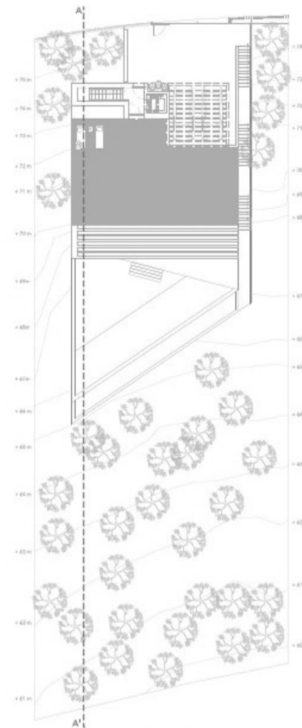
PLANTA ACCESO . IMPLANTACIÓN EN LA PARCELA. E:1/200
