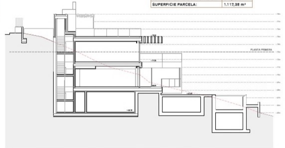
SECCIÓN AA' 11/100
