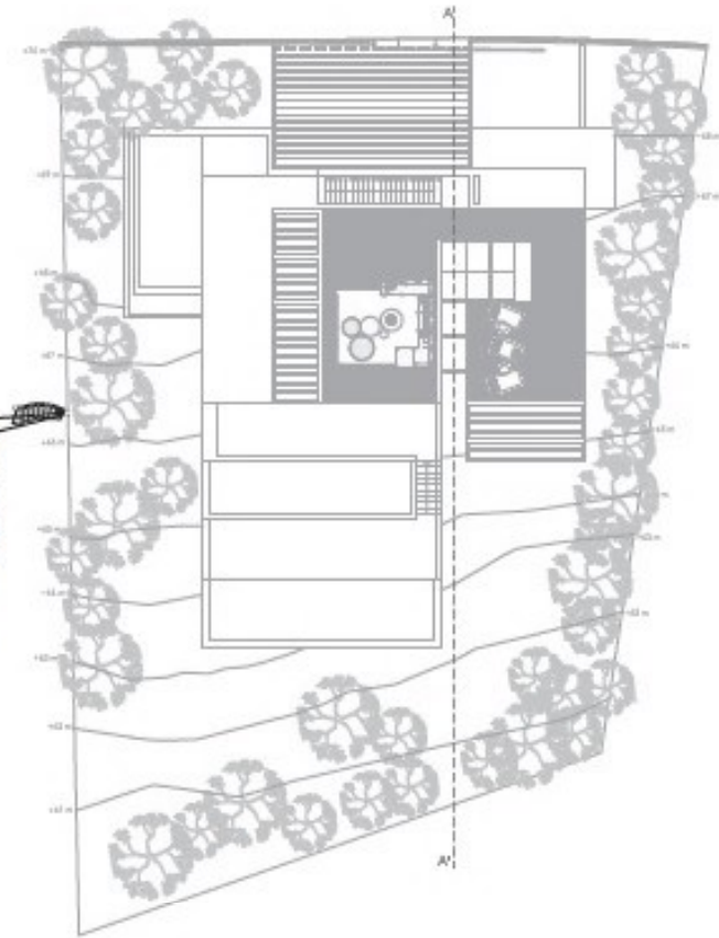
PLANTA DE CUBERTAS . EMPLANTACIÓN EN LA PARCELA 2.1/200
