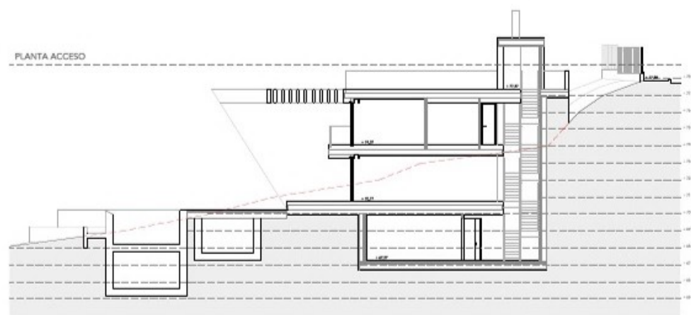
SECCIÓN A-A' 1:1/150
