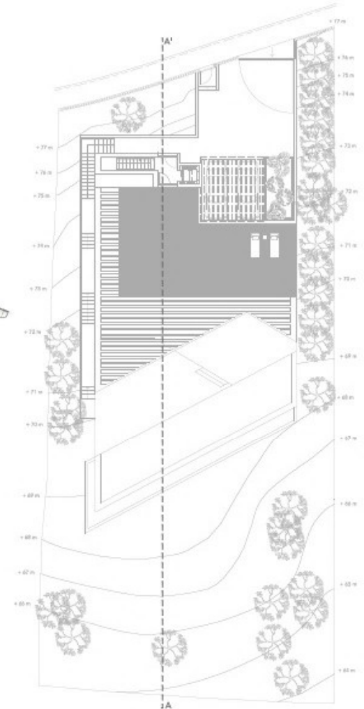
PLANTA ACCESO . IMPLANTACIÓN EN LA PARCELA. E:1/200
