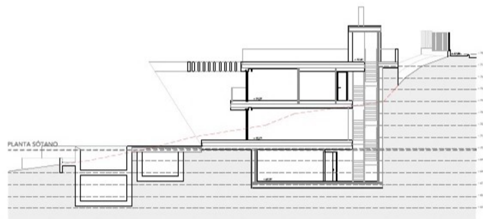
SECCIÓN A-A' E:1/150
