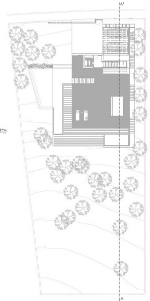
PLANTA DE CUBIERTAS - IMPLANTACIÓN EN LA PARCELA. E:1/200
